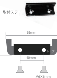
CGA09-GBR
