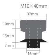
BA12-10-GBR-SET
