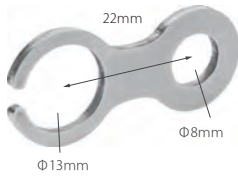
汎用ボタンスイッチφ13mm 対応 プラケット
