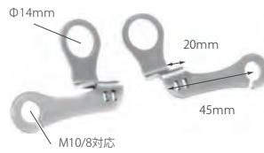
汎用ウイナーステー オフセット
