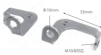
汎用ウイナーステー M10/8 対応 フォークステム用
