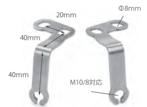
汎用ウイナーステー L-アングル 40X40 M10/8 対応
