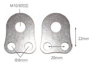
汎用ウイナーステー ストレート M10/8 対応
