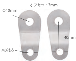
汎用ウイナーステー サスペンションマウントタイプ M8 対応
