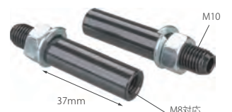
M8 ウイナーステー用 (スチール) ウイナーステーエクステンション=37mm
